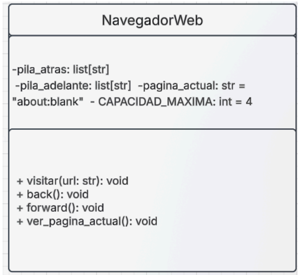
(Diagrama UML)
